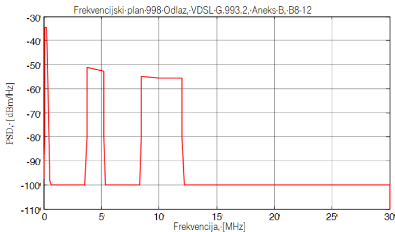
Slika 4.8.5 Maska PSD za VDSL2 frekventijski plan 998, B8-12 odlaz (crveno)
